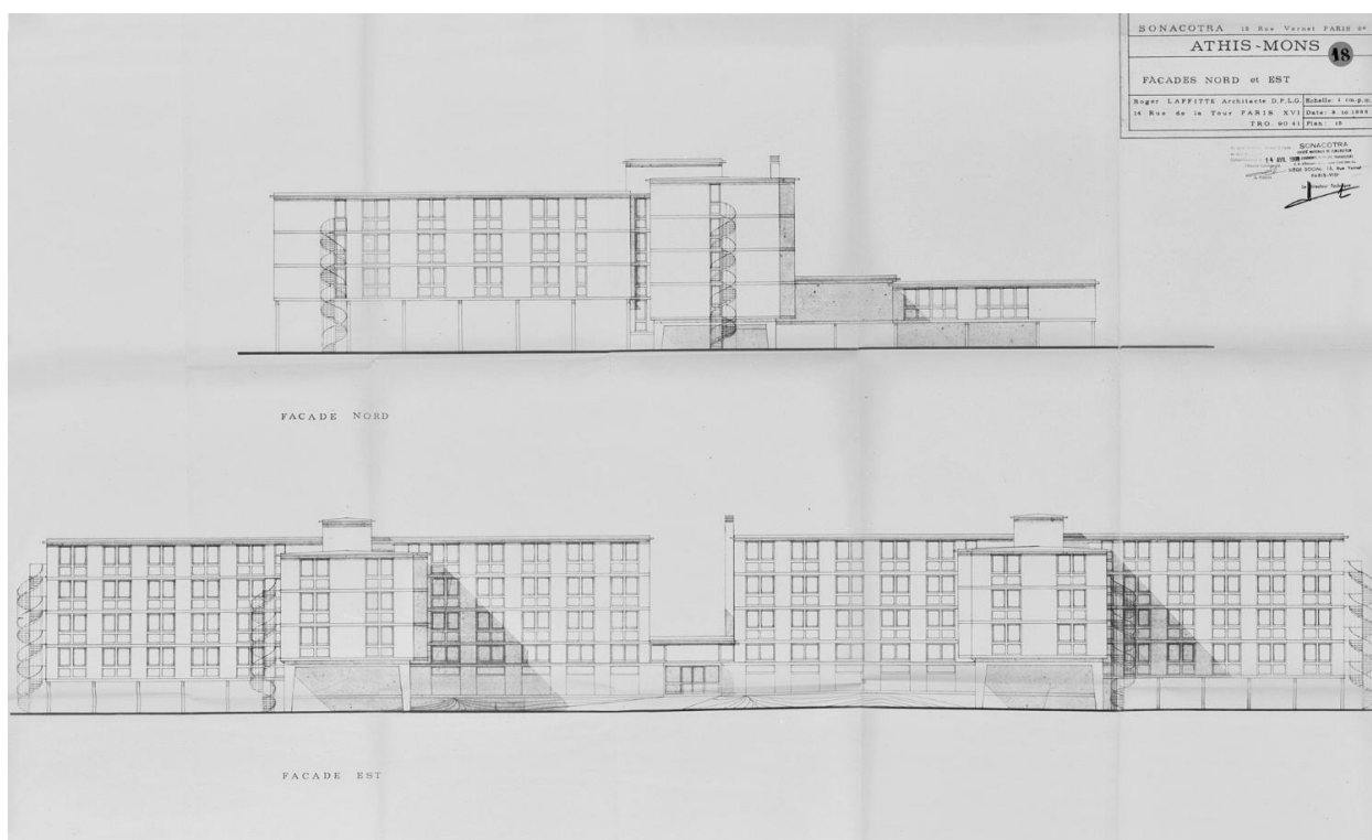
Façades nord et est ; 8 octobre 1968.
