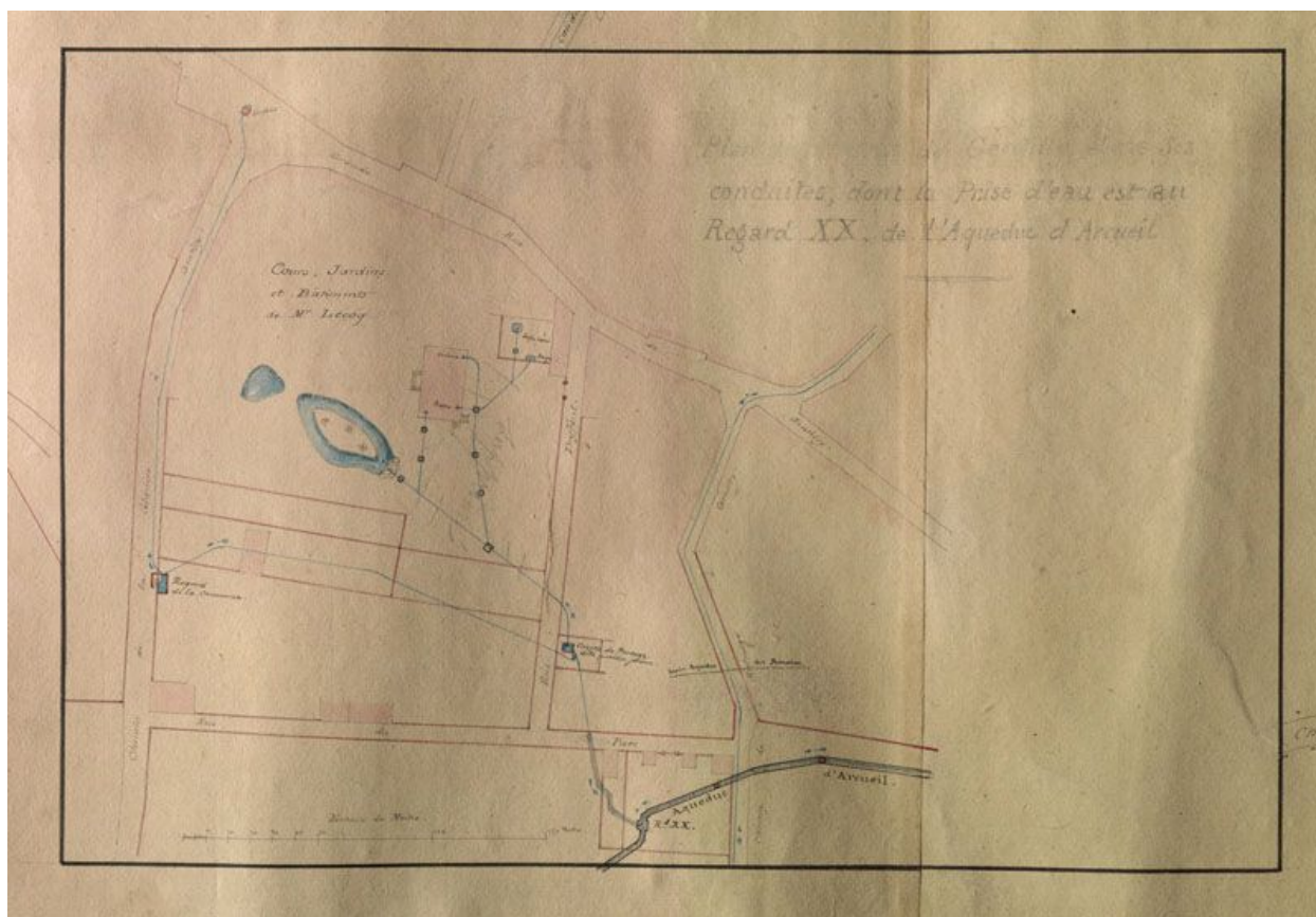
Gentilly. Plan détaillé de l'aqueduc Médicis vers 1860 : Regard XX à Gentilly. (Archives de Paris, Plan n°2522)
