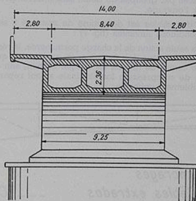
FIG. 3. — Coupe transversale du tablier.
