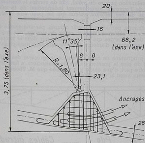
FIG. 2. — Balancier en béton armé et fretté.
