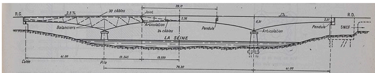
FIG. 1. — Demi-coupe et demi-élévation de l'ouvrage.
