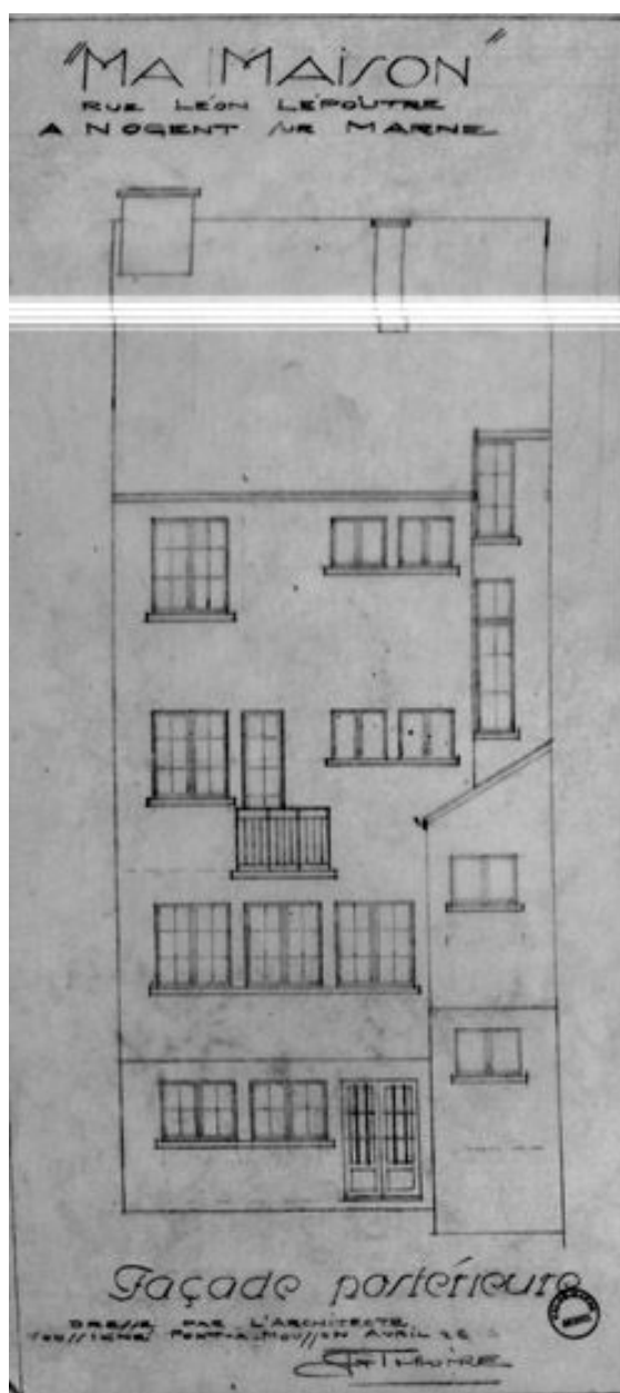
Élévation postérieure. Calque, 1926. (AD Val-de-Marne. 27 J 185)
