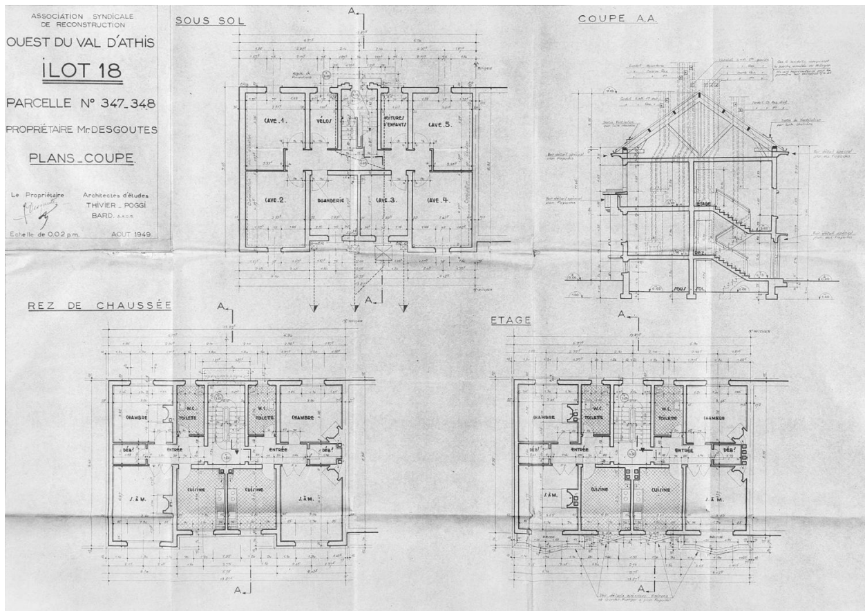
Plans et coupe de l'immeuble Desgouttes (parcelles 347-348, îlot 18, 10-10bis, rue Bertrand-Maupomé) reconstruit par Thivier-Poggi et Bard, architectes d'études, et Aubert, architecte d'opération, août 1949.
