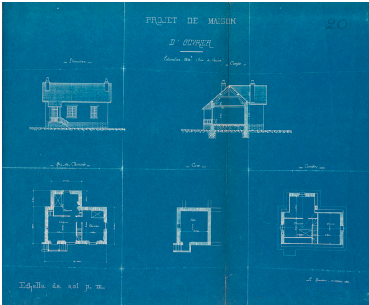
Plan. Edmond Delaire. Projet pour "le nouveau quartier" de Champagne-sur-Seine. Projet de maison d'ouvrier.
