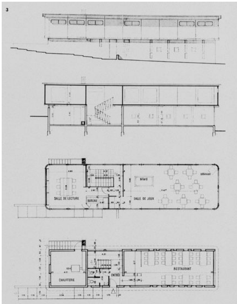
Façade, coupe et distribution. S.d. (AM Vigneux-sur-Seine)
