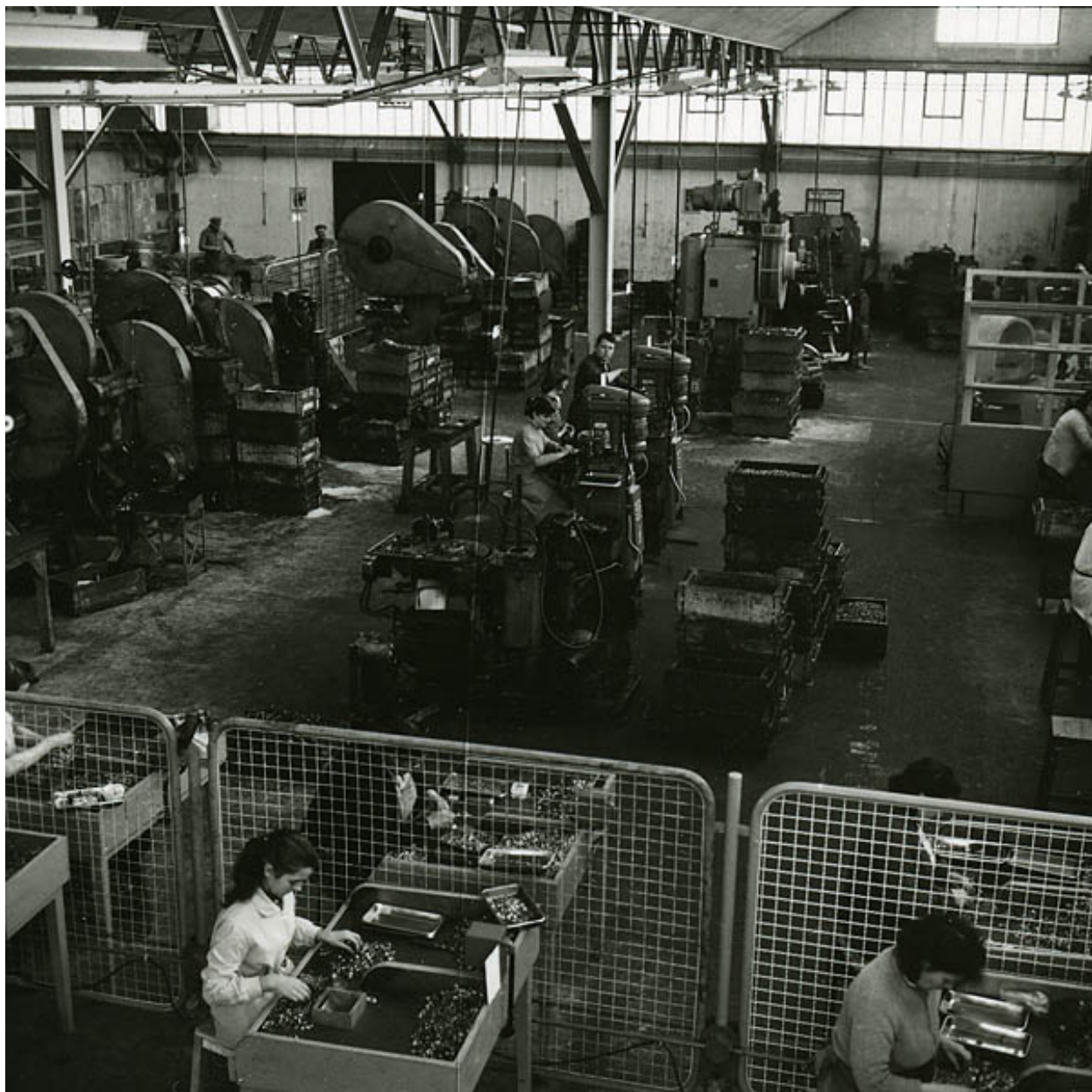
Vue intérieure de l'usine Bieth-Humbert présentant des machines à découper et emboutir et des ouvriers au travail. Photo datant des années 1950. (Collection particulière)
