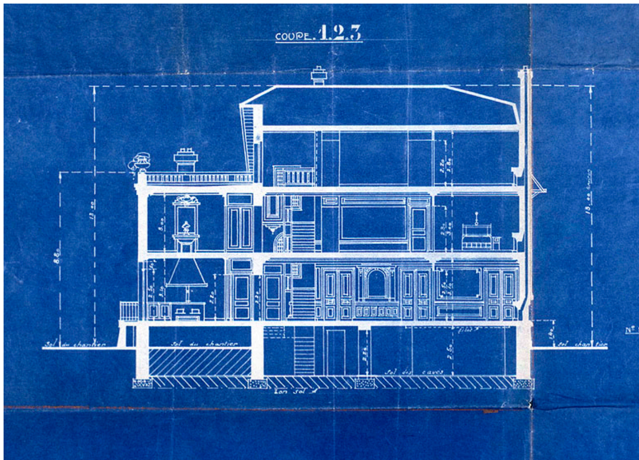
Plan bleu, maison patronale Laubeuf, coupe, 1923, archives municipales de Montreuil. (AM Montreuil)
