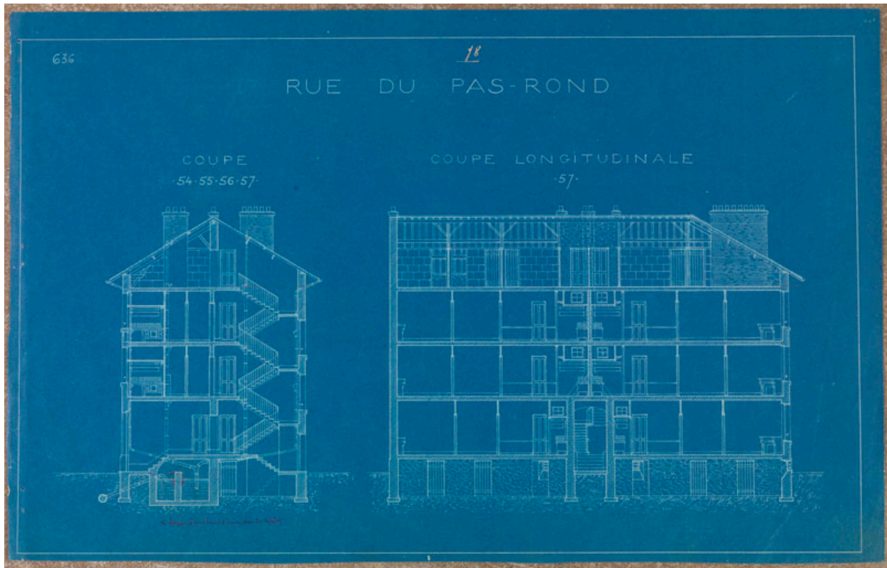
Plan. Société immobilière de Champagne. Coupe et coupe longitudinale. Rue du Pas-Rond.
