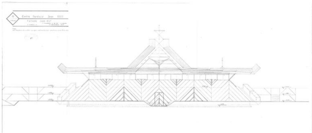
Façade sud-est.
