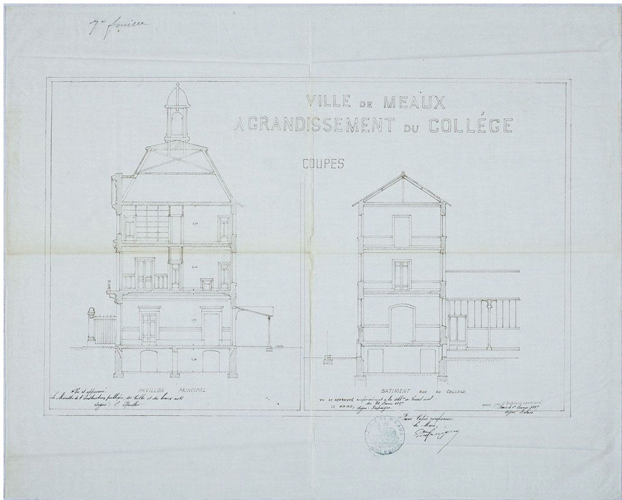
Agrandissement du collège par Delaire, 1887 : coupes. Document sur papier. (AD Seine-et-Marne. 4 Op 284/15)
