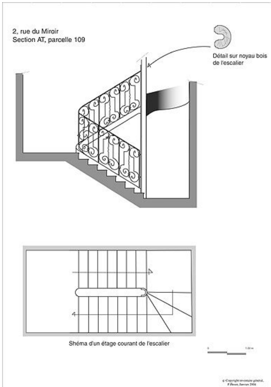
Plan et coupe de l'escalier en ferronnerie.
