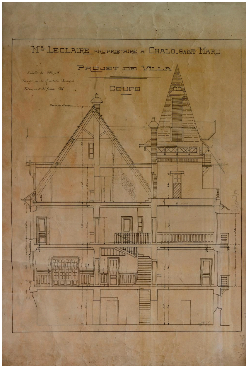
Projet de villa. Plan de coupe, daté du 22 janvier 1908
