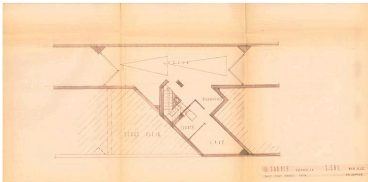
PLan du sous sol (extrait du permis de construire).
