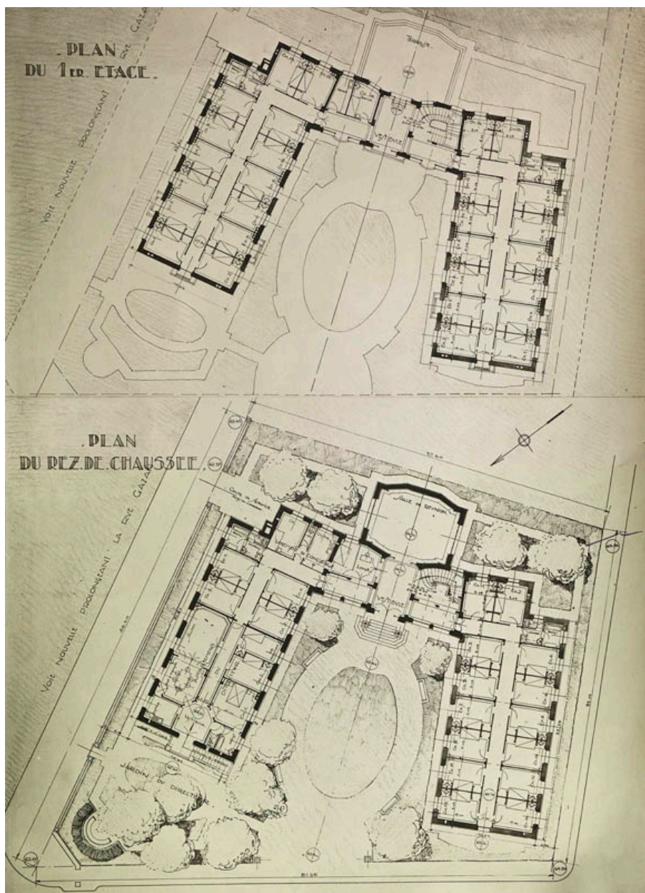
Plan du rez-de-chaussée et du premier étage, par l'architecte René Patouillard-Demoriane, s. d. Photographie. CIUP, centre de valorisation du patrimoine, P/TP-B4.
