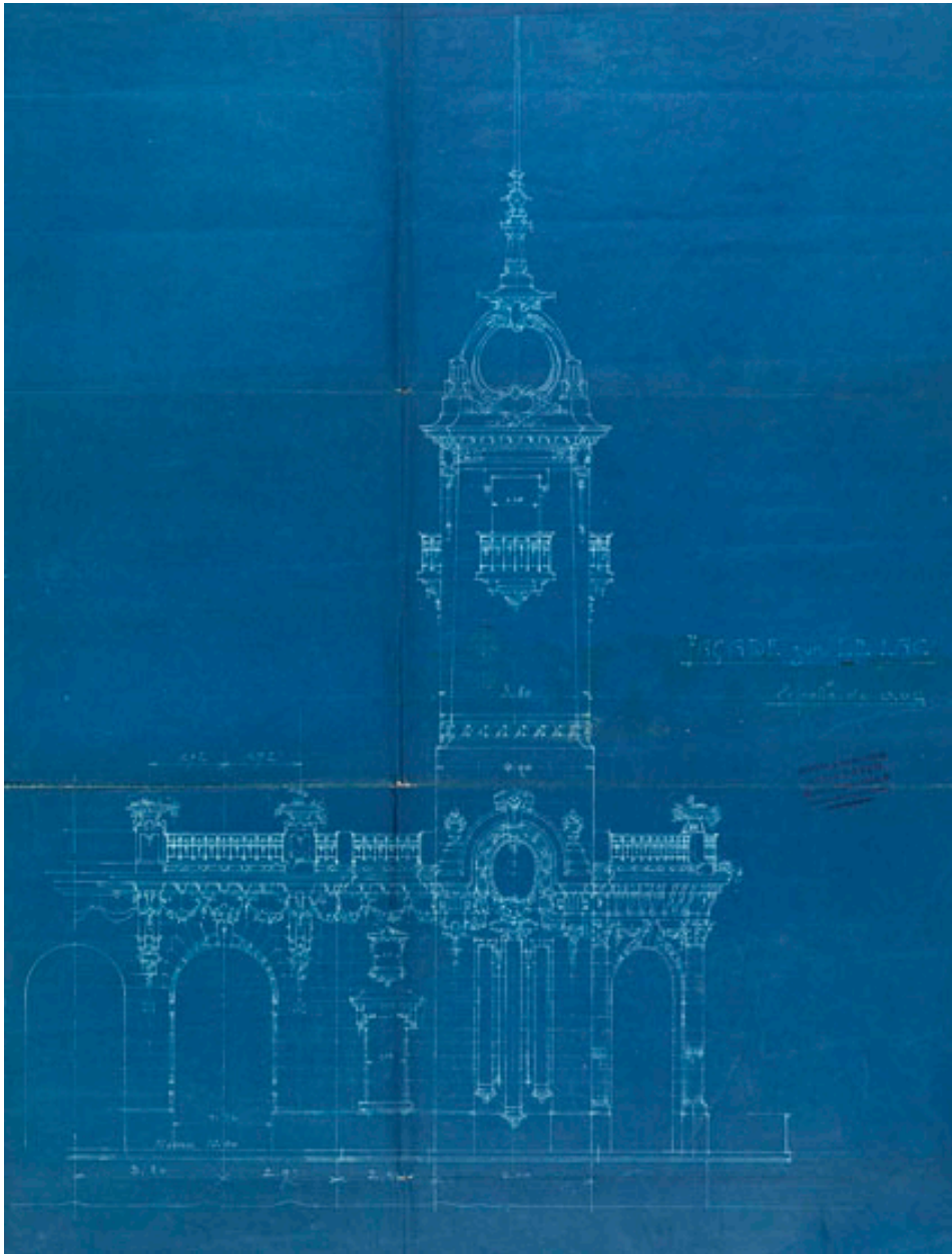
Elévation d'une façade du casino, détail sur l'une des deux tours. (AM Enghien-les-Bains, M109, plan n°20)
