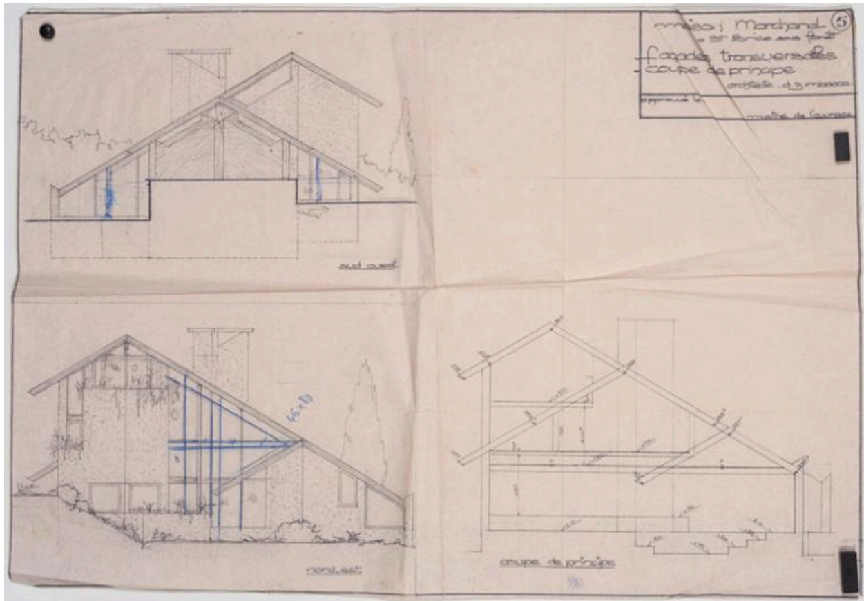
Façades transversales, Maison Marchand.
