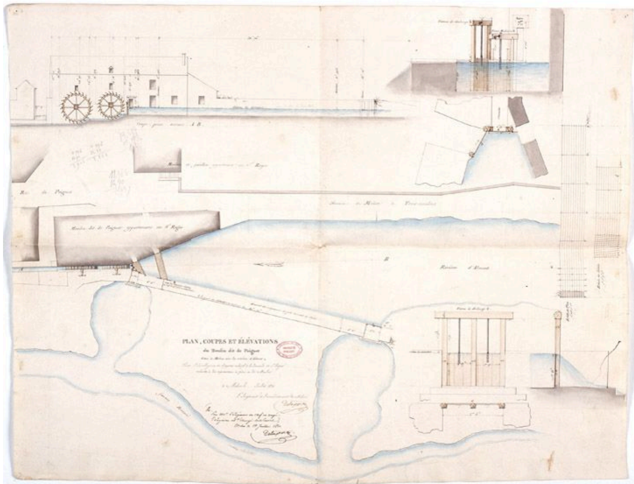
Plan, coupes et élévations du moulin de Poignet. Papier aquarellé, juillet 1821. (AD Seine-et-Marne. 3 S 3)
