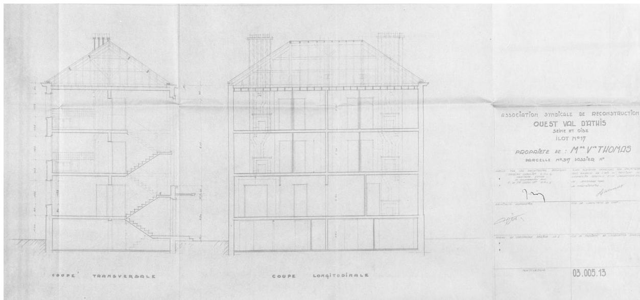
Coupes de la maison construite dans l'îlot 17, parcelle 317, pour Mme Vve Thomas, par Jacques Chauliat, s. d.
