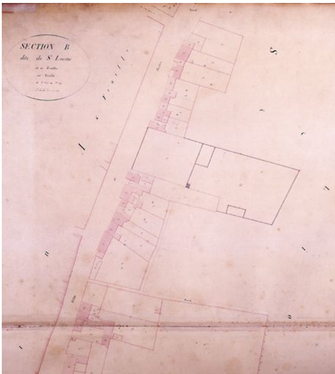
Plan parcellaire de la commune de Melun, levé en 1826 ( . ) sous la direction de M. Semane géomètre en chef, par M. Portant géomètre de première classe. Section B, dite de Saint-Liesne, 10eme feuille, 2eme partie. Papier aquarellé. (AM Melun)
