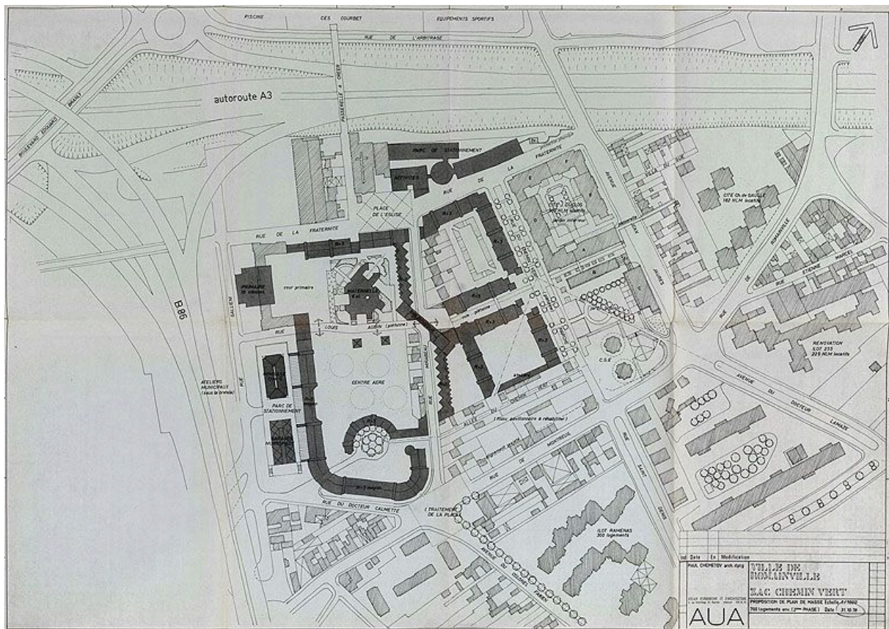
Z.A.C. du Chemin Vert. Plan de masse. (AM Romainville)
