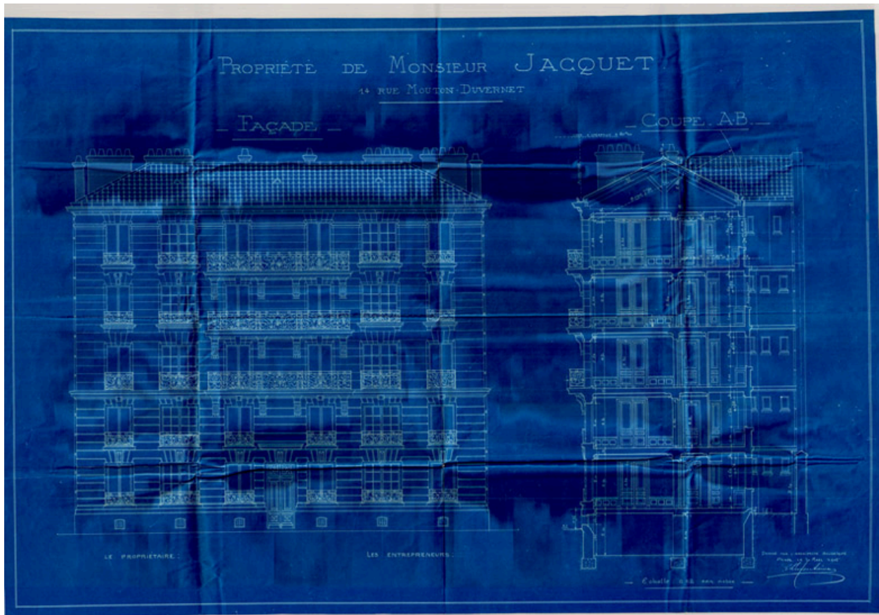
Façade et coupe.-Plan, 1905. (Archives de Paris, VO11 2486).
