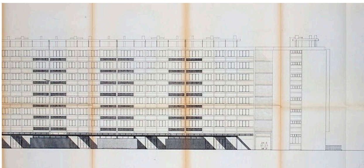
Cité dite Résidence Saint-Hubert. Plan de la façade avant d'un bâtiment donnant sur la place en U.
