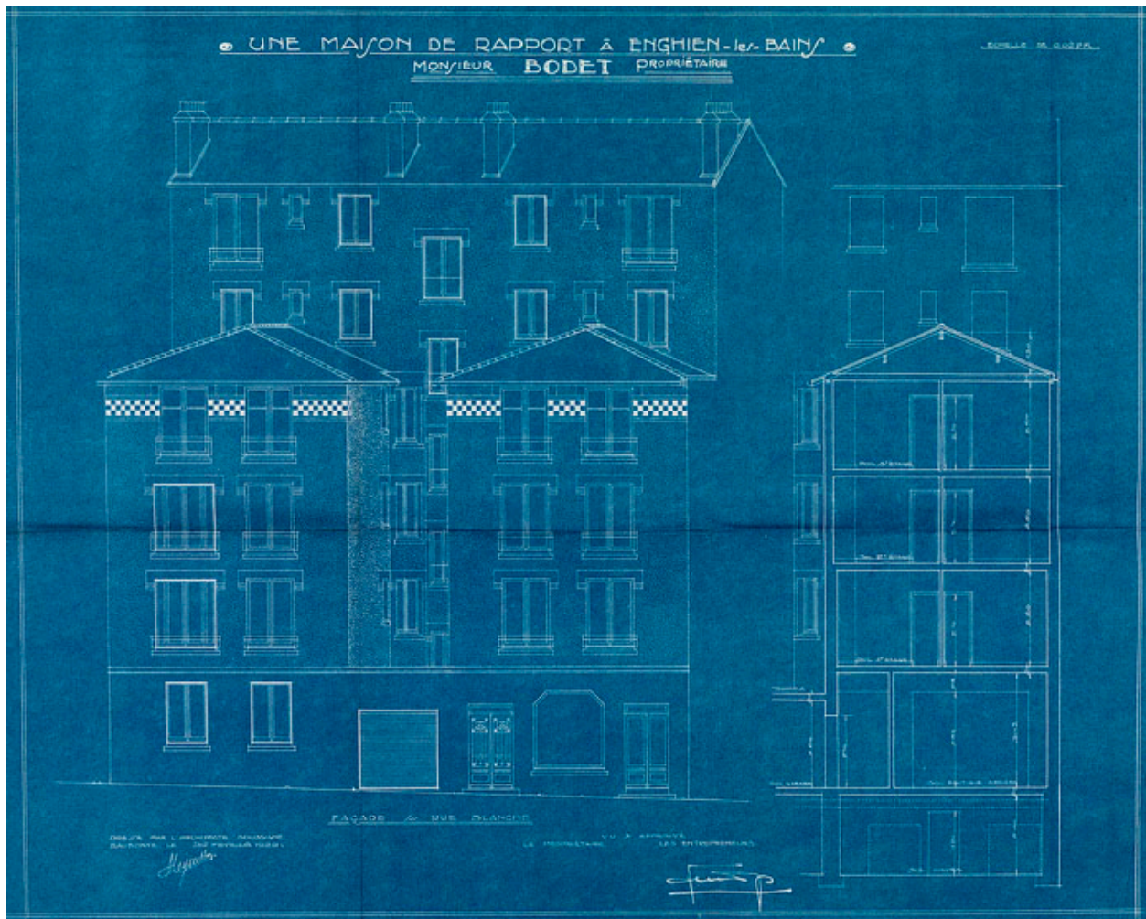
Élévation et coupe d'un immeuble construit pour monsieur Bodet en 1929, rue Blanche. (AM Enghien-les-Bains, Fonds des autorisations de permis de construire)
