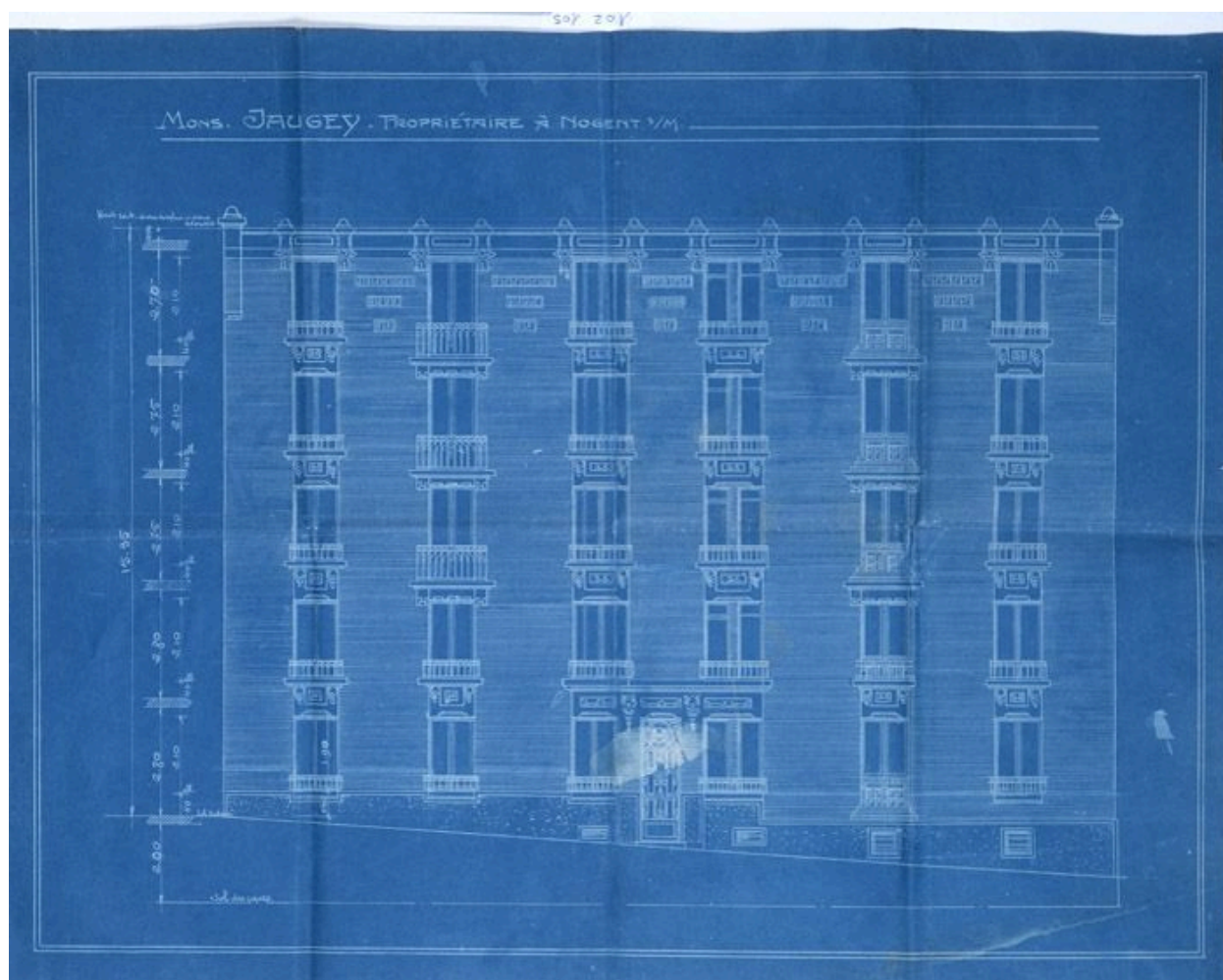
Plan de demande d'autorisation de construire un immeuble pour Mr Jaugey, non localisé. Elevation. Signé Nachbaur. 1913. (AM Nogent-sur-Marne. 1 02 105)
