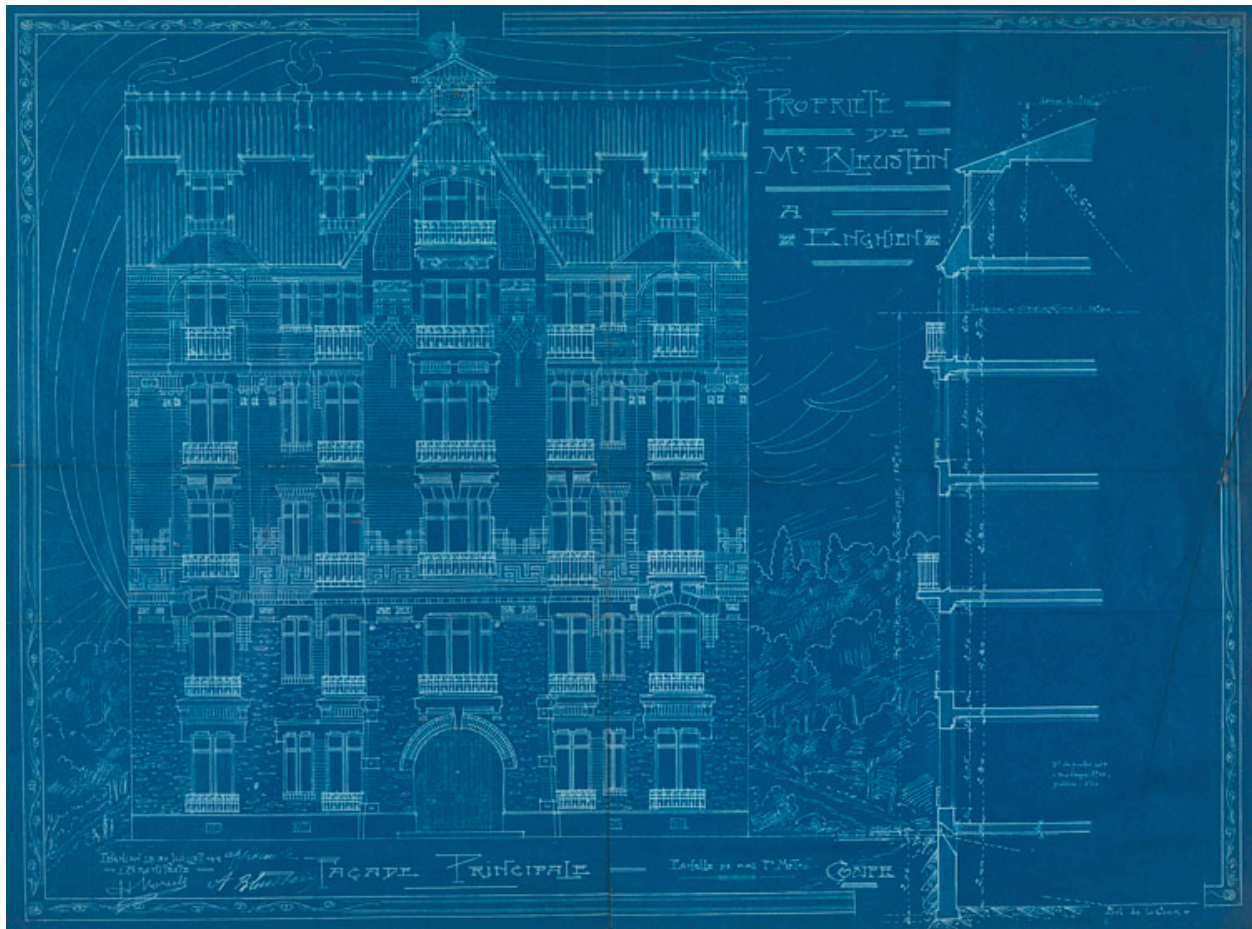
Élévation de la façade sur rue, deuxième projet : l'ensemble a quatre niveaux plus un étage de comble. (AM Enghien-les-Bains, 1T 95)
