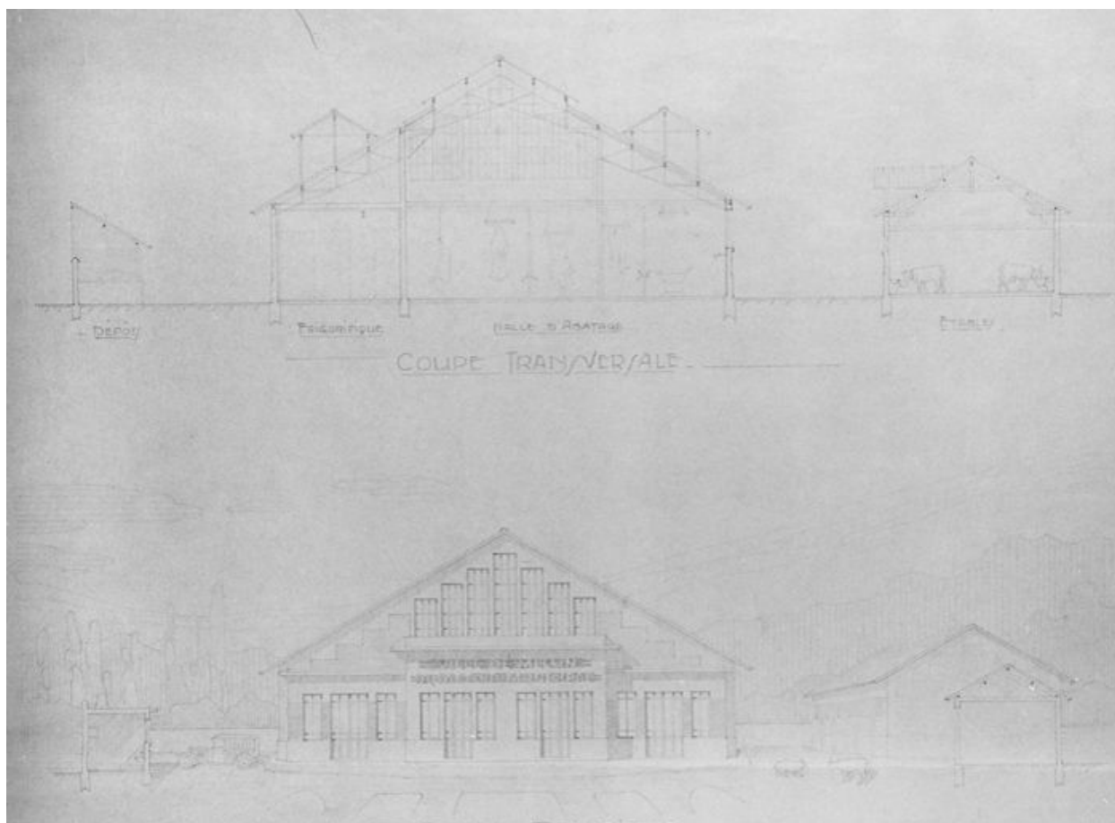
Ville de Melun. Projet de construction d'un nouvel abattoir. Coupe transversale, façade principale. 1/100e. Papier, tirage d'architecte, 1930 (janvier). (AM Melun. 1 Fi 786)
