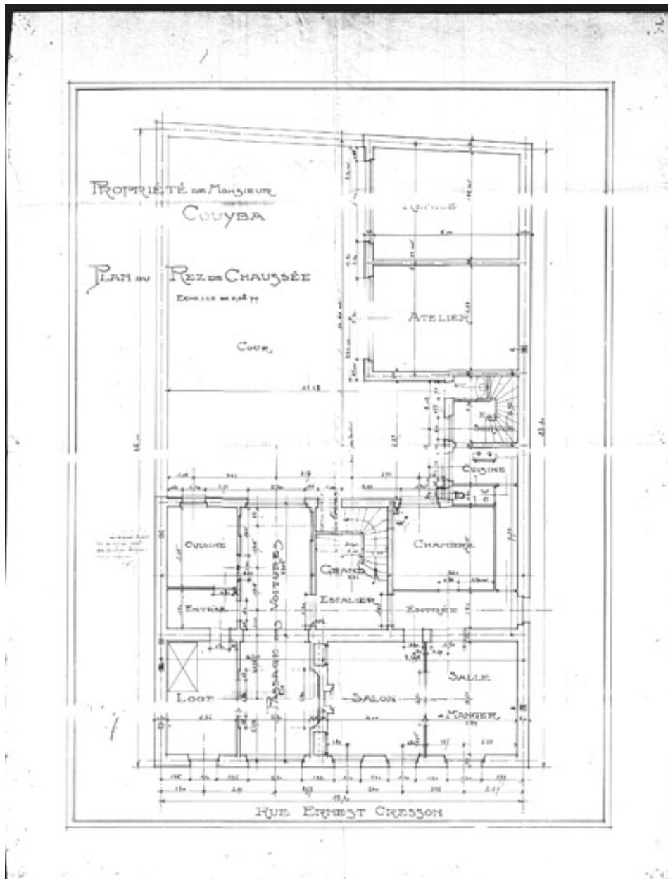
Rez de chaussée du 18 rue Ernest Cresson, propriété de M.Couyba. -Plan. (Archives de Paris, VO11 1131).
