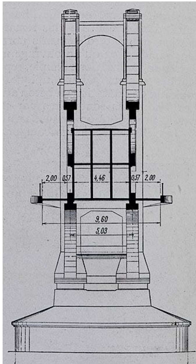
Ivry-sur-Seine, Charenton-le-Pont. Passerelle industrielle d'Ivry-Charenton. Coupe schématique sur une pile. Tiré de : Travaux, juillet 1939, p. 280.
