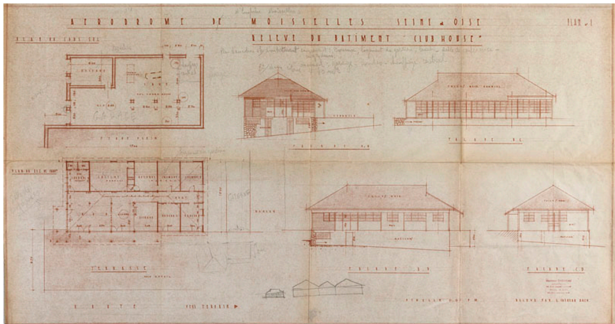
Plan et élévation des bâtiments vers 1937. (AM Enghien-les-Bains)
