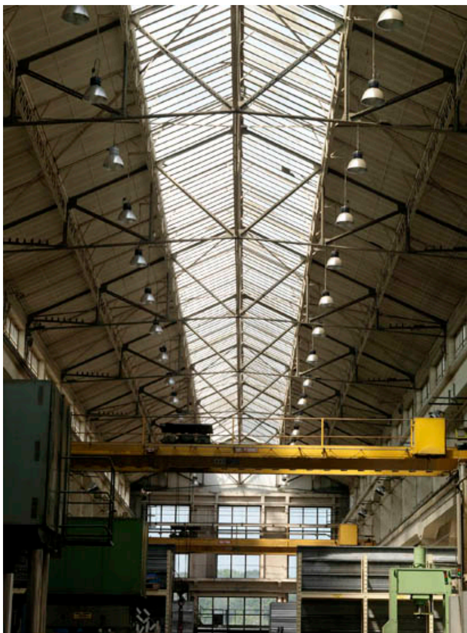
Vue intérieure. Liaison longitudinale nord. Ateliers d'armement puis de mécanique (1918). Actuellement entreprise Jeumont Electric. La verrière et la charpente métallique.
