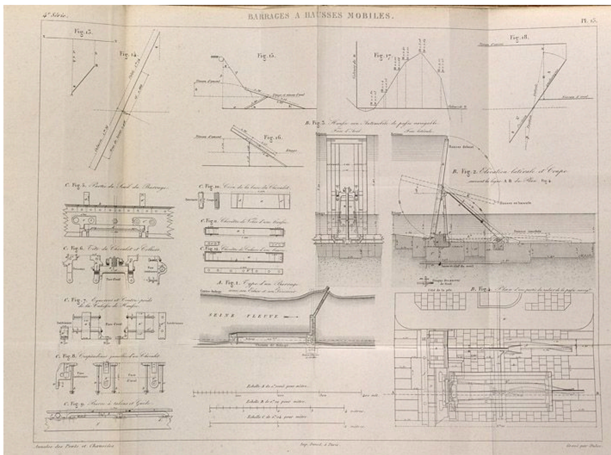
Barrages à hausses mobiles. Elévations et coupes. Tiré de : Mémoire sur les barrages à hausses mobiles / M. Chanoine et M. de Lagrené. In Annales des Ponts et Chaussées, 2e semestre, 1861, n° 21, pl. 15-17.
