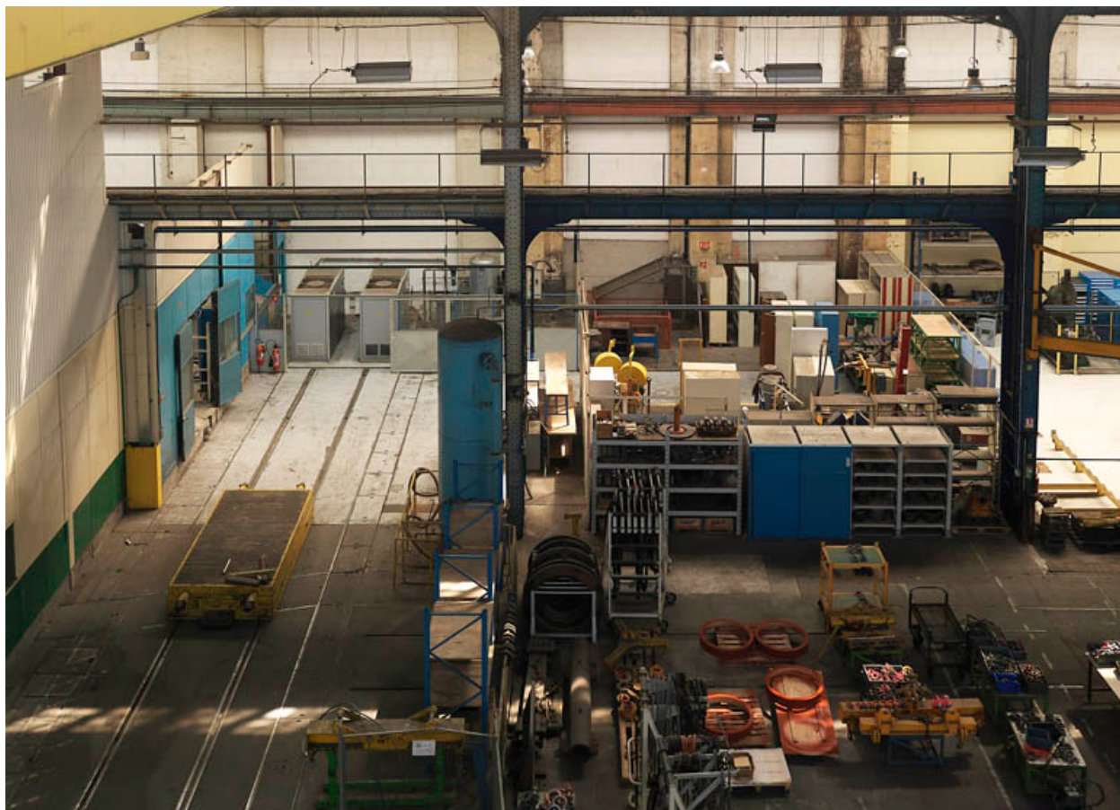
Vue intérieure de la nef centrale. Montage, machines-outils (1901-1903). Actuellement entreprise Jeumont Electric.
