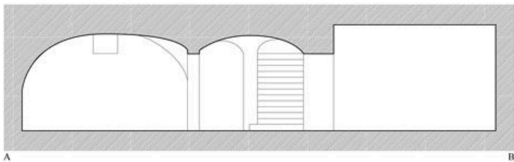
Coupe AB
