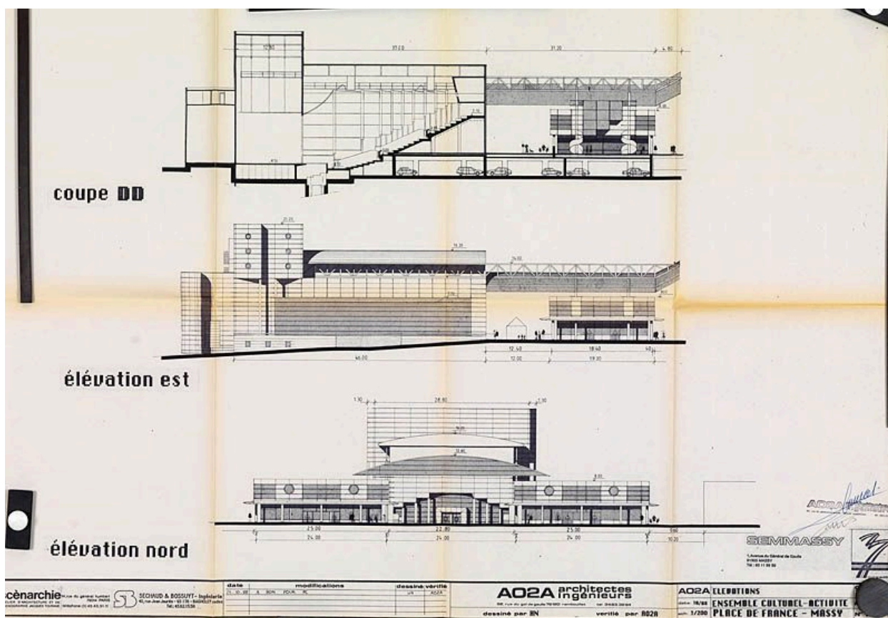
Elévations de l'opéra. (AM Massy)
