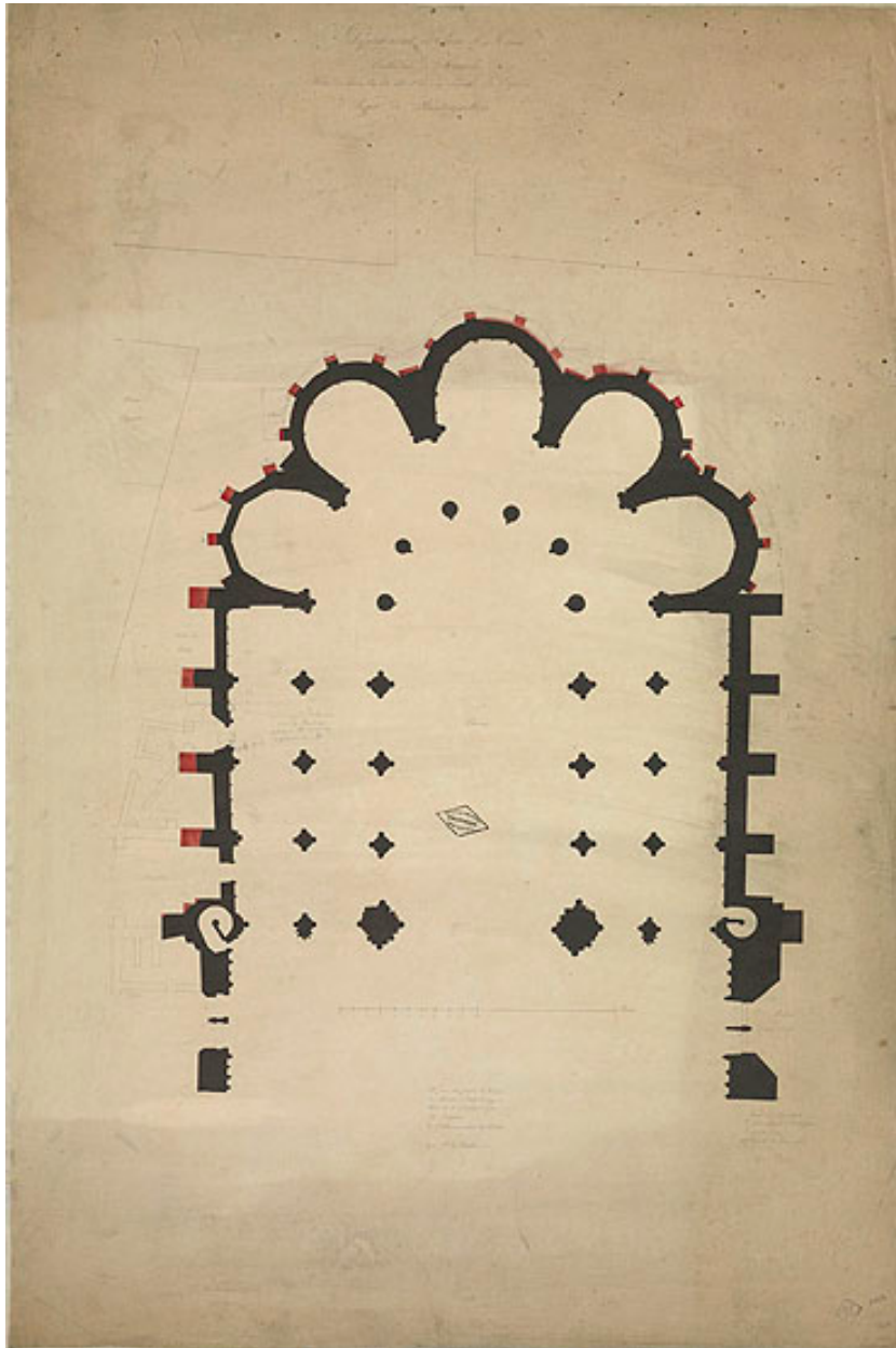
Plan du choeur et du chevet avec indication des travaux, par Danjoy (13 juin 1850). Encre sur papier, 13 juin 1850. (Médiathèque de l'architecture et du patrimoine. 0082/077/1014, document n° 081837.)
