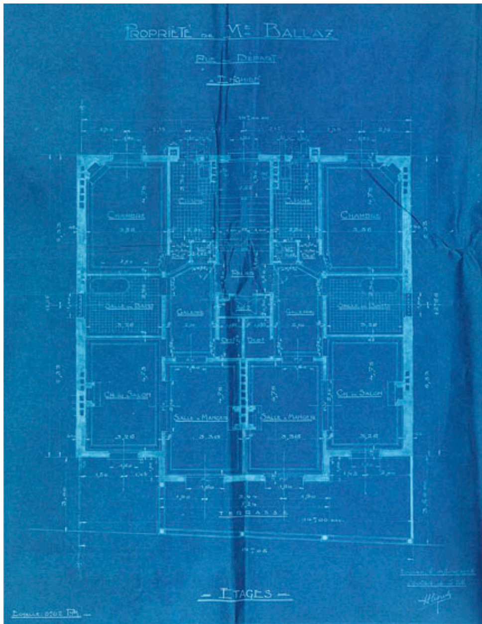
Plan du premier étage avec terrasse (1926). (AM Enghien-les-Bains, 1T 66)
