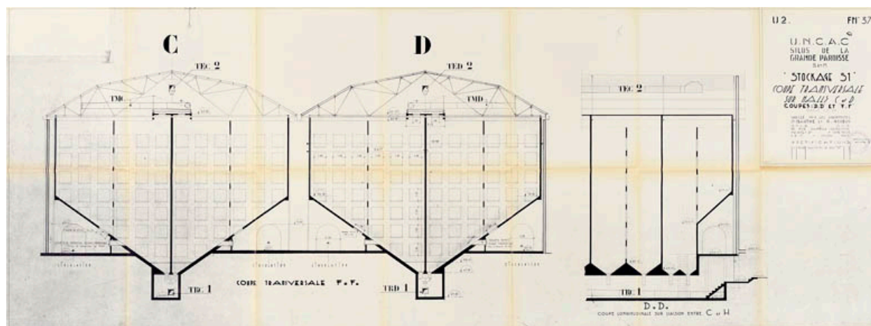
Silos de l'UNCAC de la Grande Paroisse. Stockage S1. Coupe transversale sur halls C et D. Dressé par les architectes P.Barthe et R.Robin, 15 septembre 1955. (Archives départementales).
