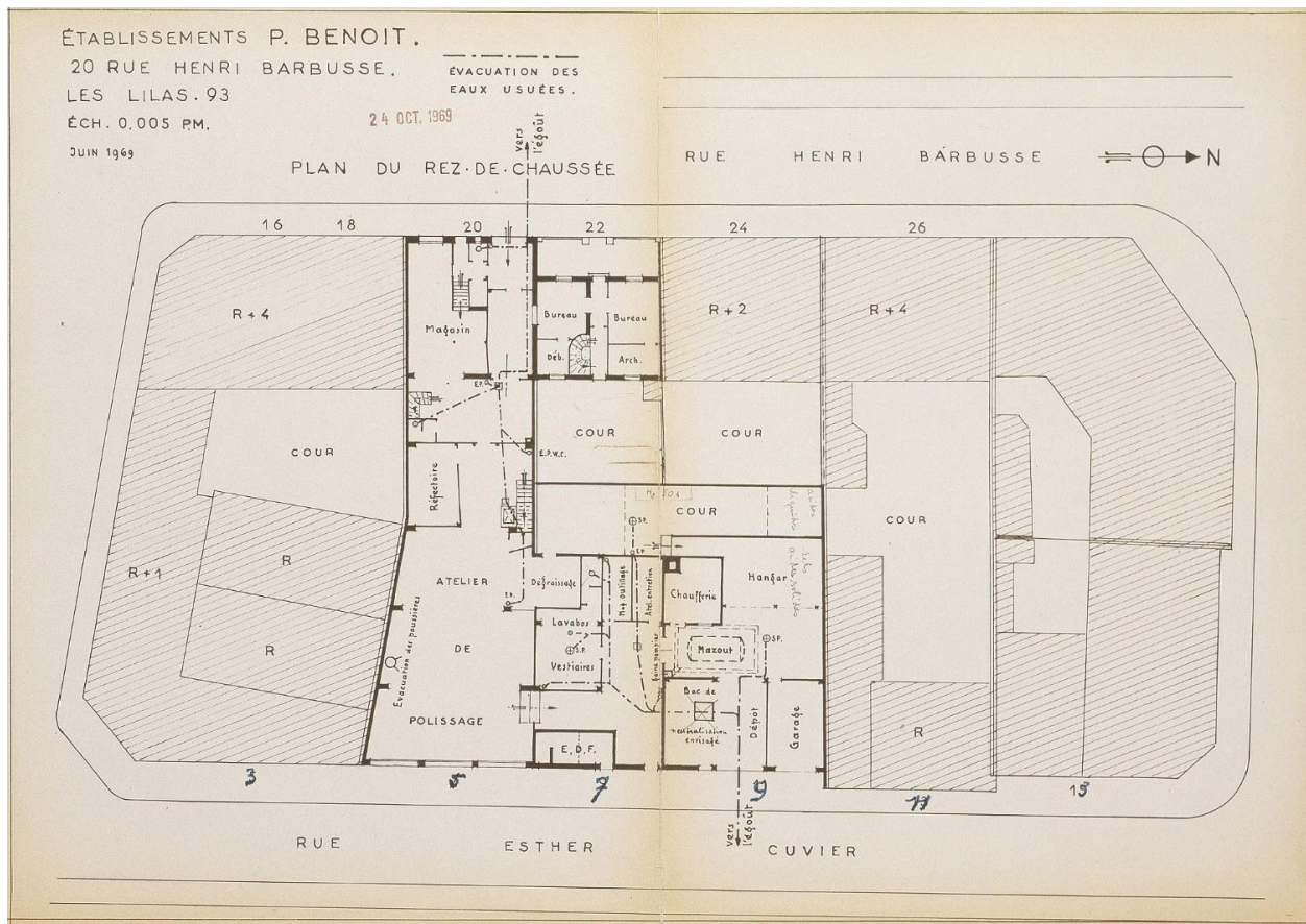
Plan du rez-de-chaussée, indiquant la fonction des ateliers, 1969 (AD93 1322 W 242).
