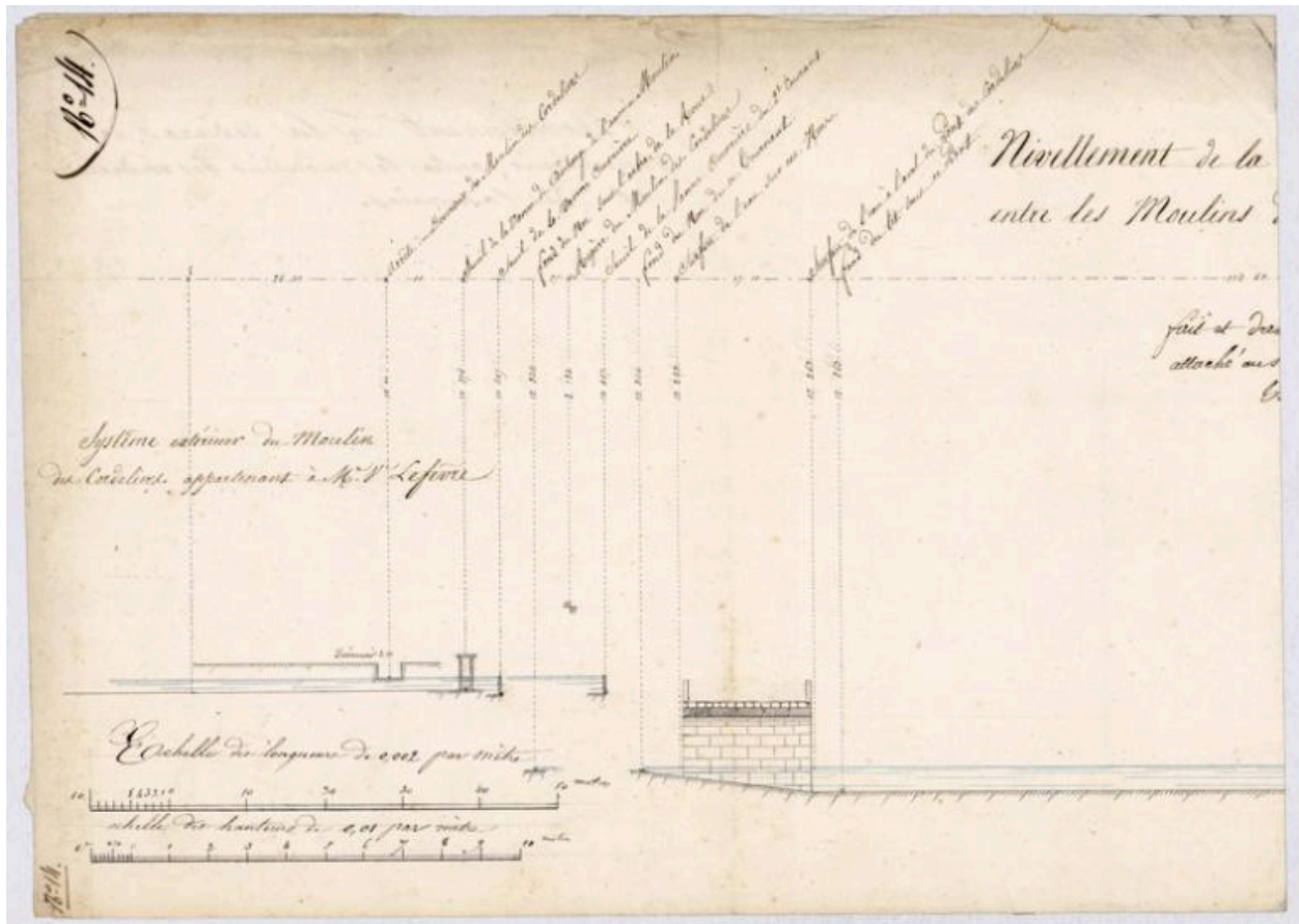
Nivellement de la Vaucoleurs en 1830. Partie gauche. (AD78 7s 285)
