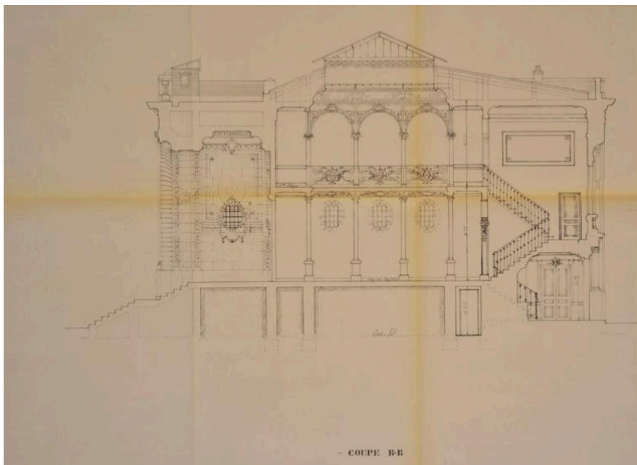
Coupe longitudinale. Projet de restauration en 1981. Tirage. (AM Mantes-la-Jolie 53 W 123)
