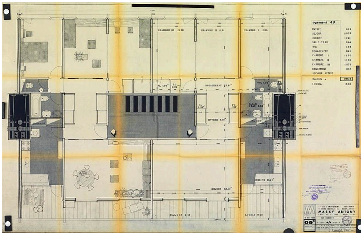
Plan de cellule 4 pièces, 14 mai 1963. (AM Massy, 7 T 74)
