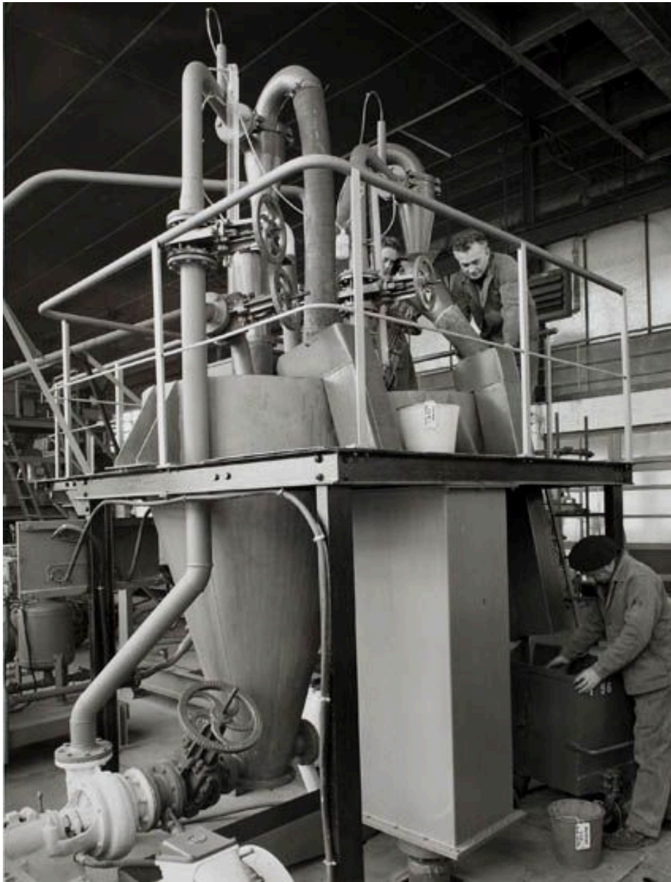
Vue intérieure de la station d'essai. Photographie. (AD Seine-et-Marne, 256J3)
