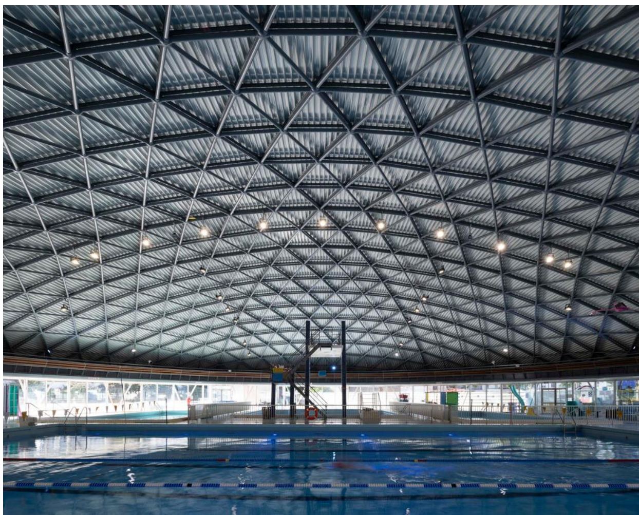
Stade nautique de Drancy. Charpente métallique.
