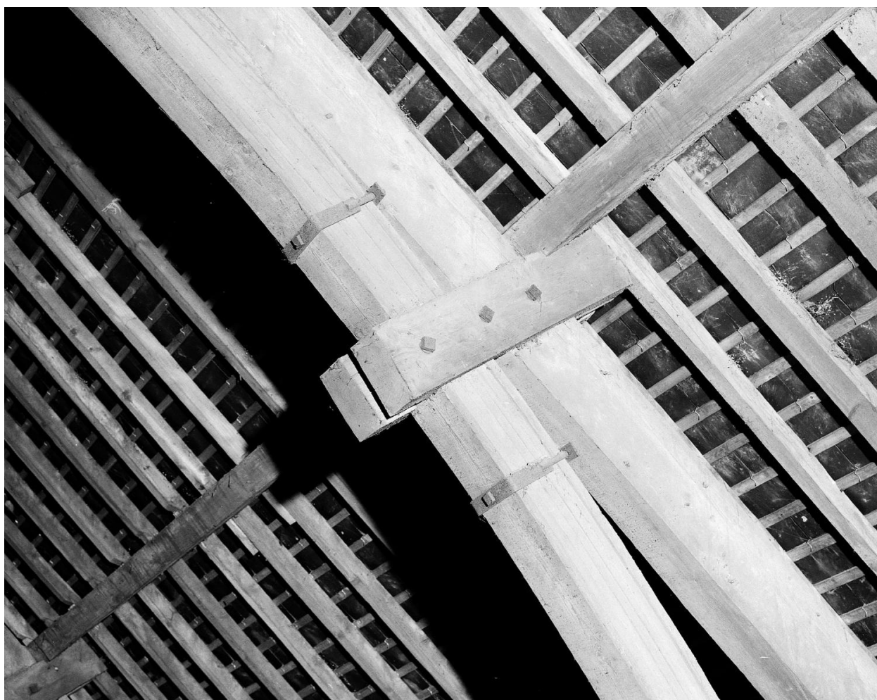
Charpente : détail du liaisonnement blochet-arbalétrier.
