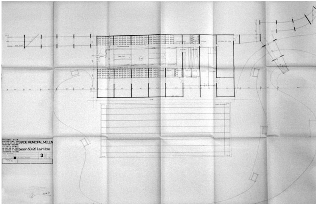
Bassin découvert : plan au niveau des vestiaires. Tirage d'architecte, 14 octobre 1966. (AM Melun. 466 W 84)
