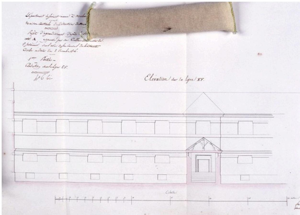
Projet d'extension par Solente, architecte départemental : élévation selon la ligne EF. Papier aquarellé, 1816-1818. (AD Seine-et-Marne. 1 Y 52)
