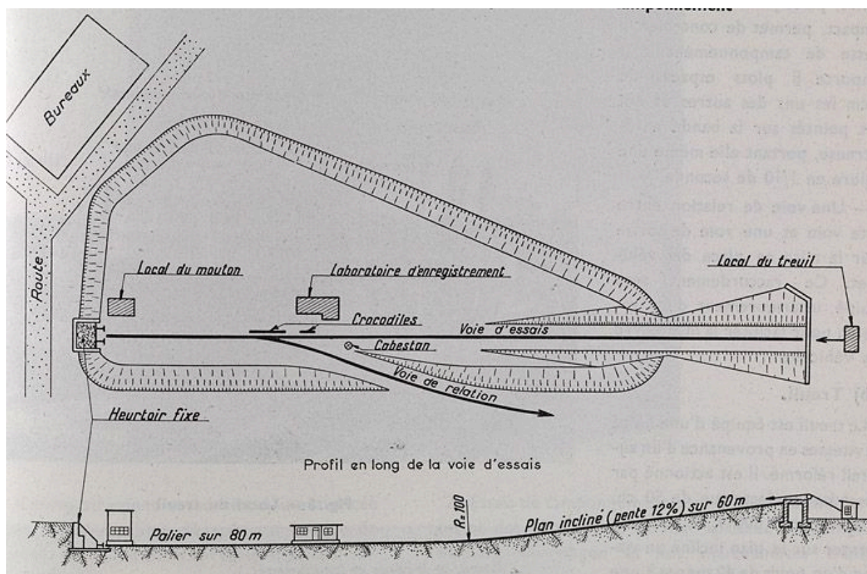
Vitry-sur-Seine, station d'essais ferroviaires. Profil en long de la voie d'essais. Tiré de : Revue générale des chemins de fer, juin 1959.
