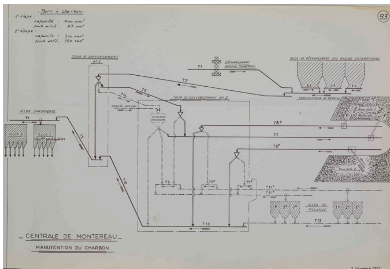
Schema de la manutention du charbon dans le parc a charbon.
